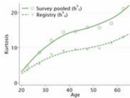
(d) Kurtosis
