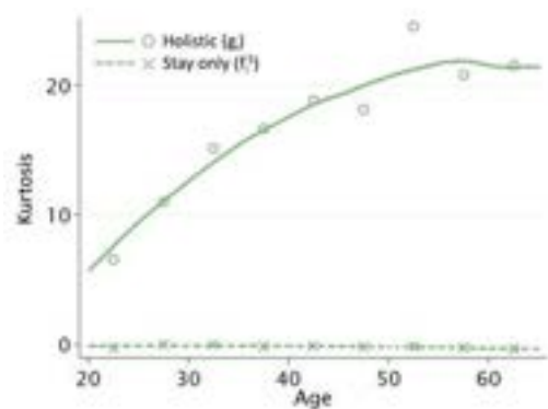
(d) Kurtosis
